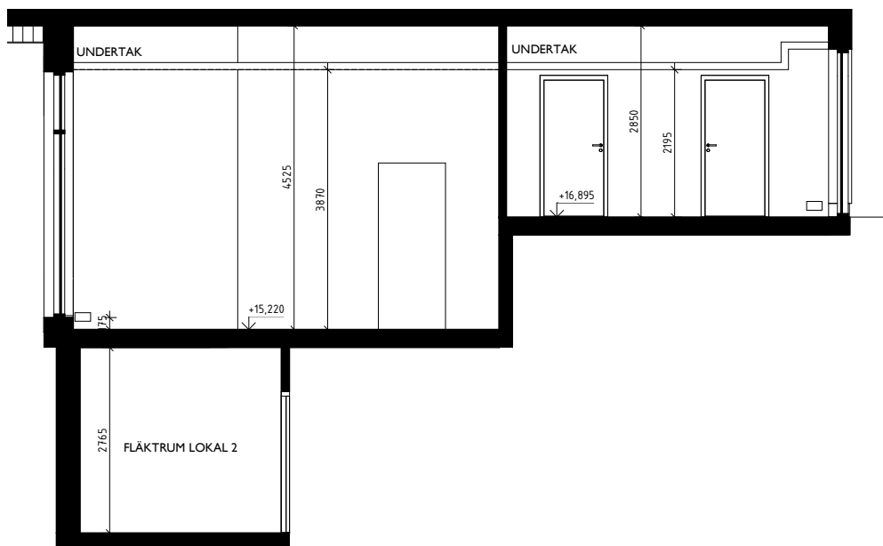
Lokal 2 C-C
