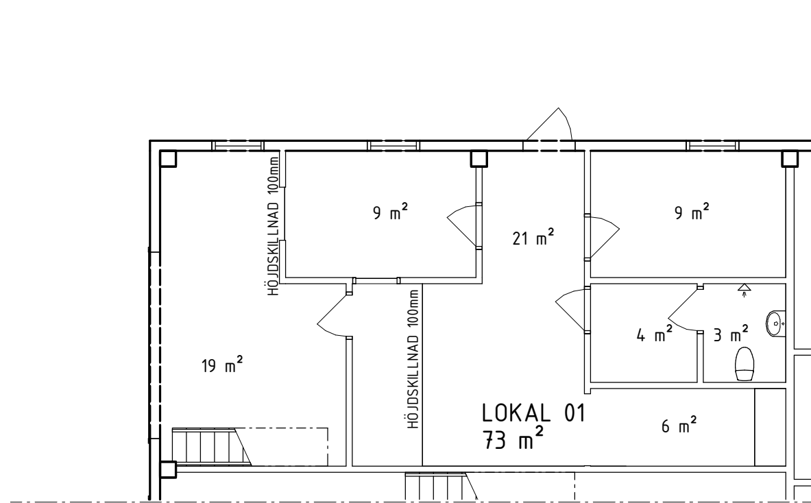
LOKAL 01
