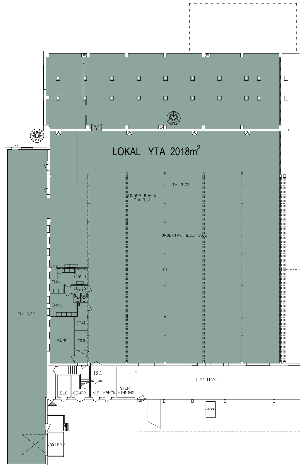
PLAN 0 SKALA 1:300 i A3
