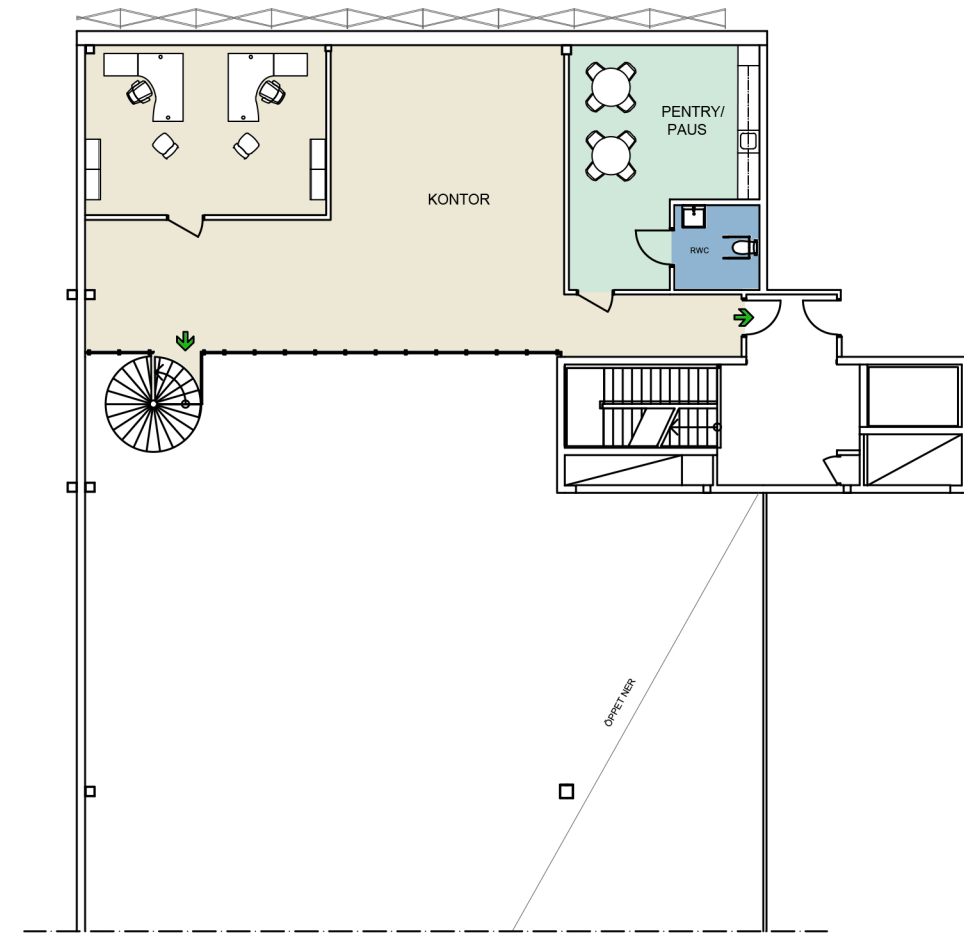
Entrésolplan Kontor
