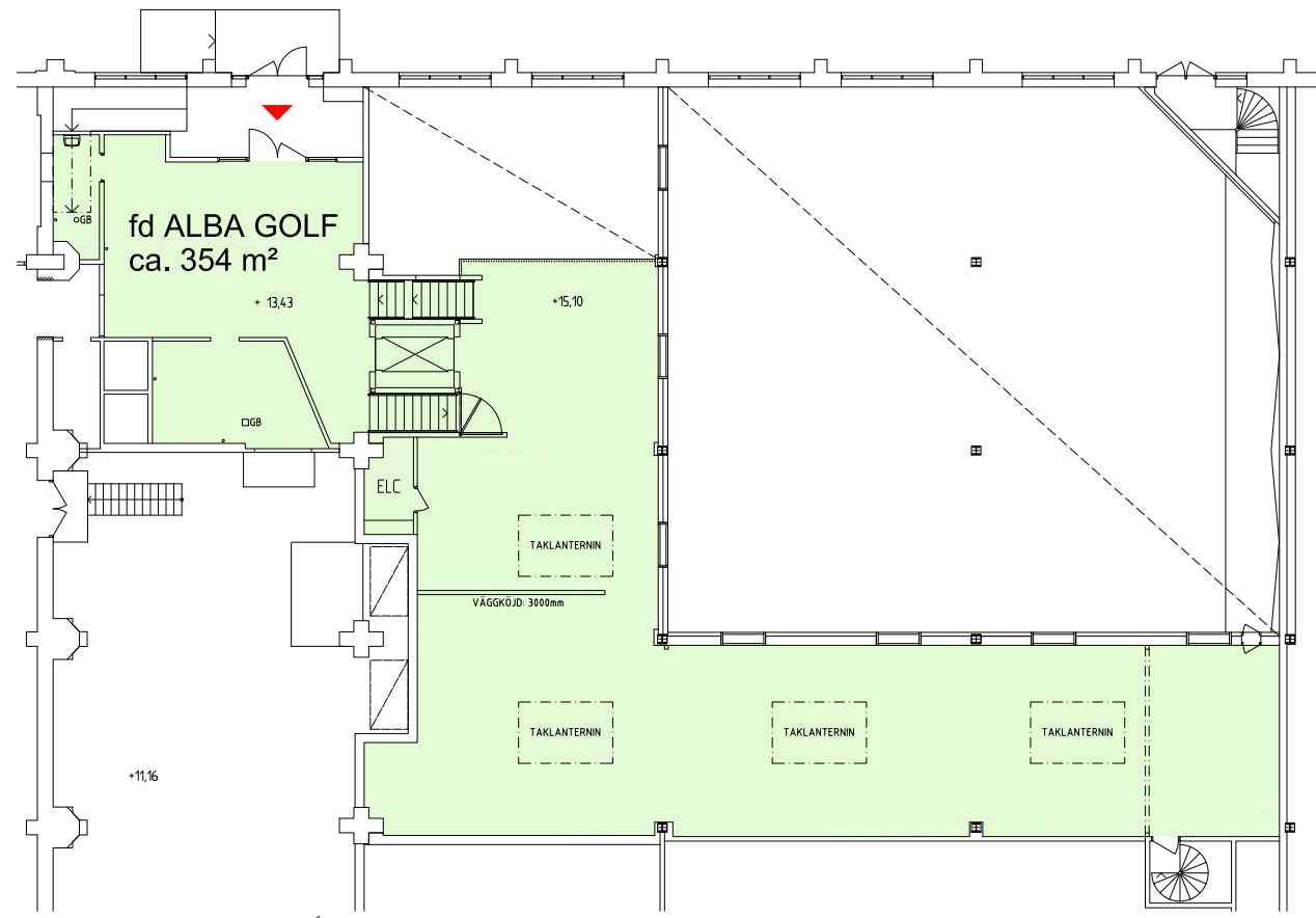
PLAN 2, +13.43(ENTRÉPLAN)/+ 15.10
