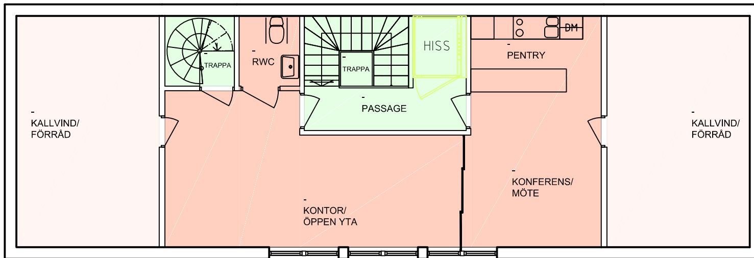
PLAN, VÅNING 3
