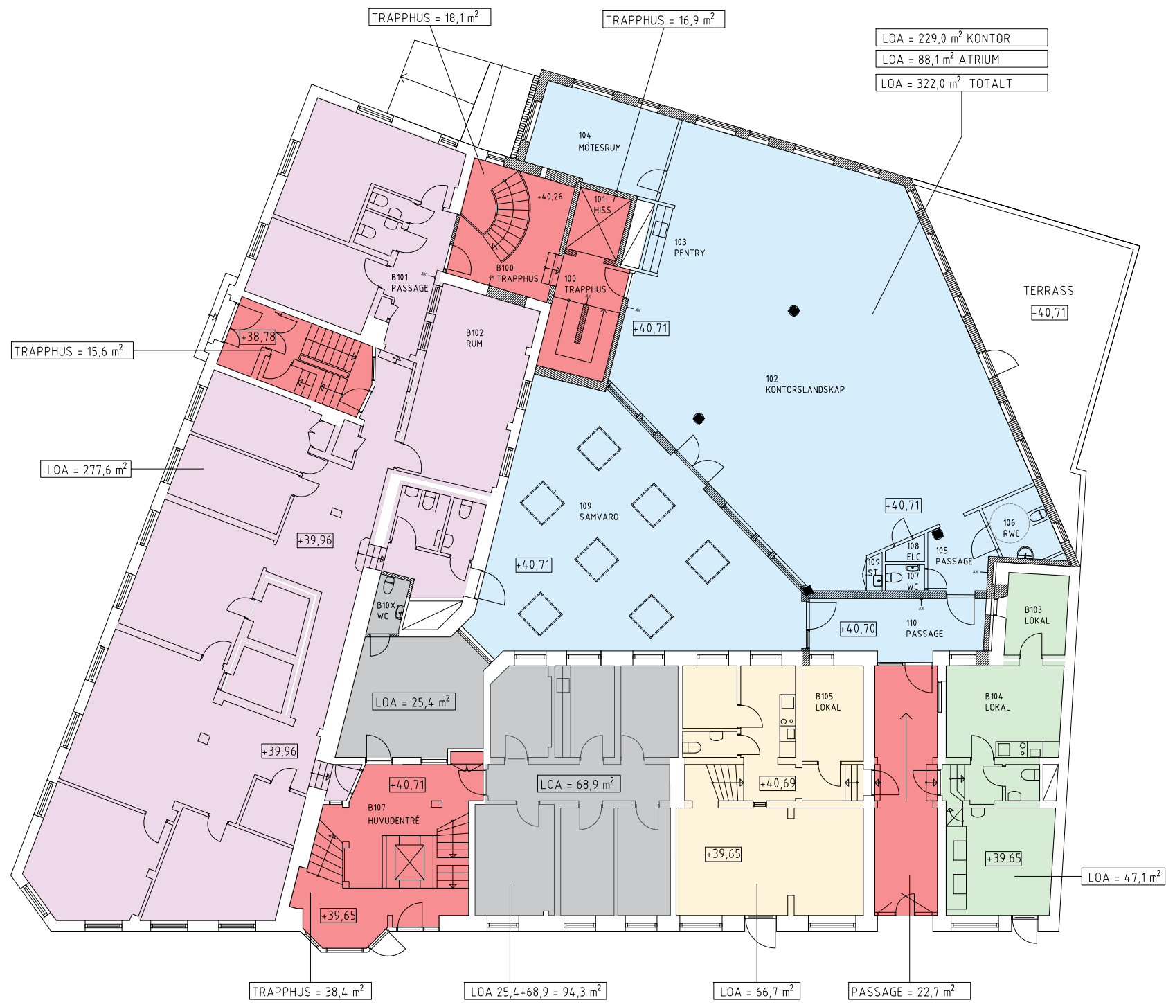
PLAN 1 / BOTTENVÅNING
