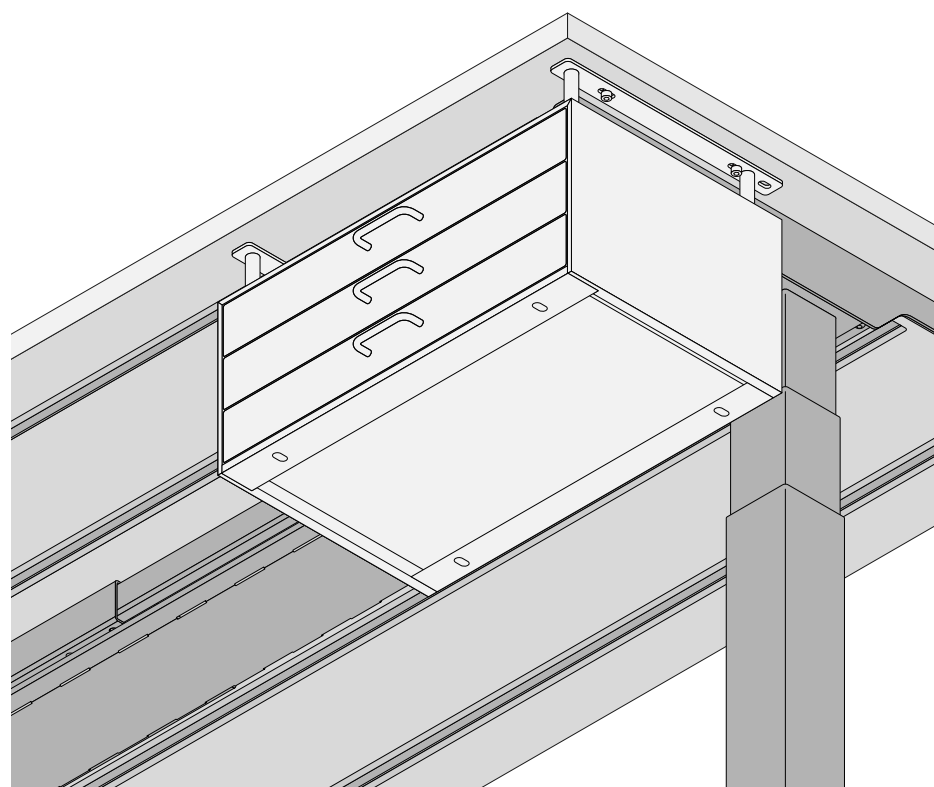
設置タイプ B FlexiSpot のサポートプレートを跨いで レール2本と外側のネジ穴で固定する ・ Base Slider × 2 (別売)
