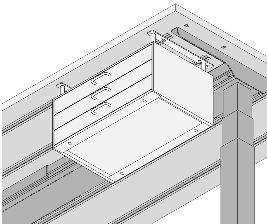
設置タイプ A レール2本で固定する ・ Base Slider × 4 (別売)
