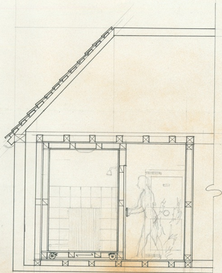
① SECTION 1:20
