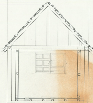
② SECTION 1:20
