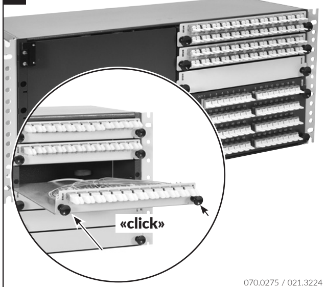
G6 Unterhalt / Service
