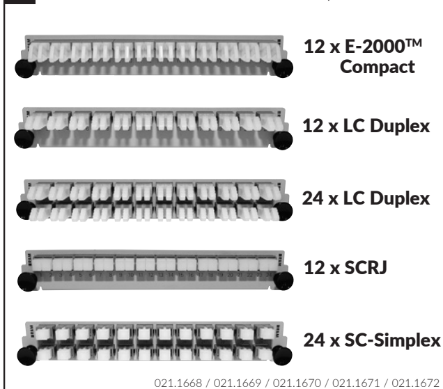
G2 Max. 6 Patch Einschübe / Max. 6 patch inserts
