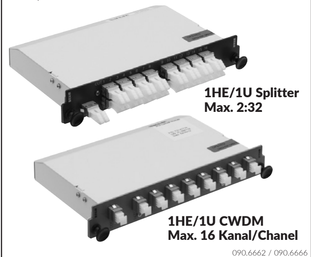
G3 Splitter & xWDM Einschübe (1HE - 3HE) / Splitter & xWDM inserts (1U - 3U)
