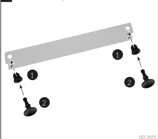
G1 Blindabdeckung / Blind cover
