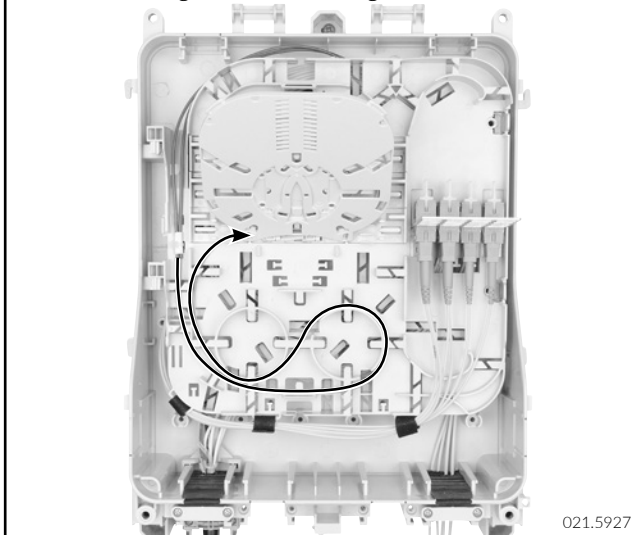
F4 Inlay - fiber routing Fasereinlage - Faserführung
