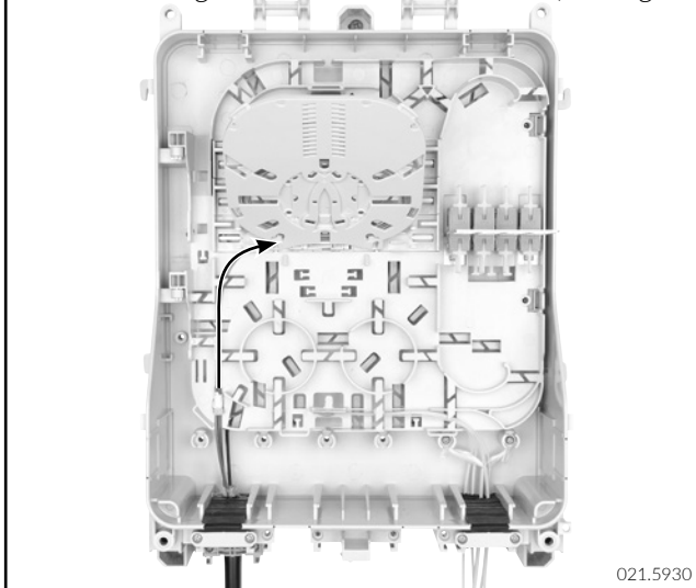
F6 Inlay in lower position - fiber routing Fasereinlage in unterer Position - Faserführung
