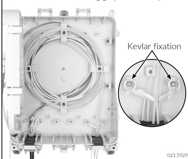
F7 Optional spliced dropcable application Alternative Anwendung gespleisstes Dropkabel
