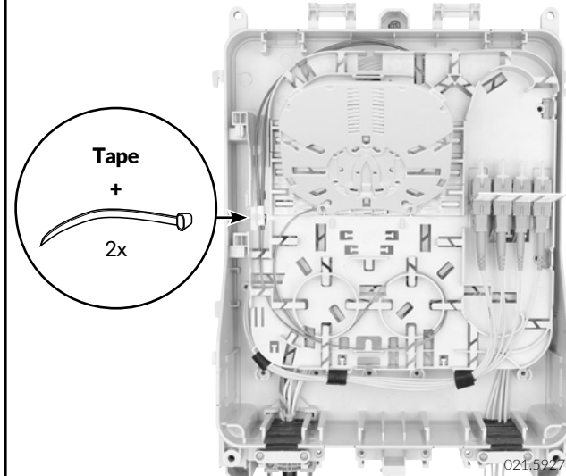
F3 Fixation of loose tubes Befestigung der Bündeladern
