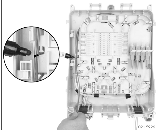
F2 Mark and strip the loose tubes Markieren und abisolieren der Bündeladern
