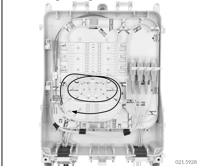
F5 Inlay - fiber routing front side Fasereinlage - Einlage Oberseite
