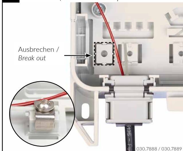
D7 Zugentlastung mit Eingangs-Kit Modular / Strain relief with cable entry kit Modular
