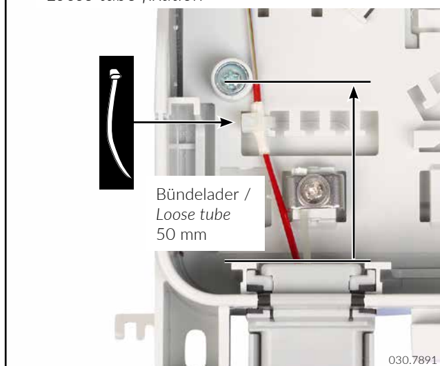
D9 Bündelader Befestigung / Loose tube fixation
