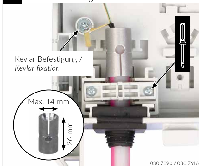
D10 Mikrorohr mit Gasblocker / Micro-duct with gas termination
