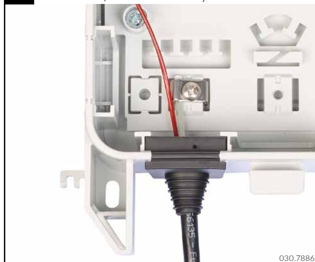
D8 Zugentlastung mit Eingangs-Kit Basic / Strain relief with cable entry kit Basic
