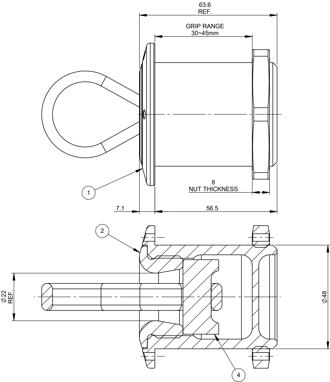
SECTION A-A
