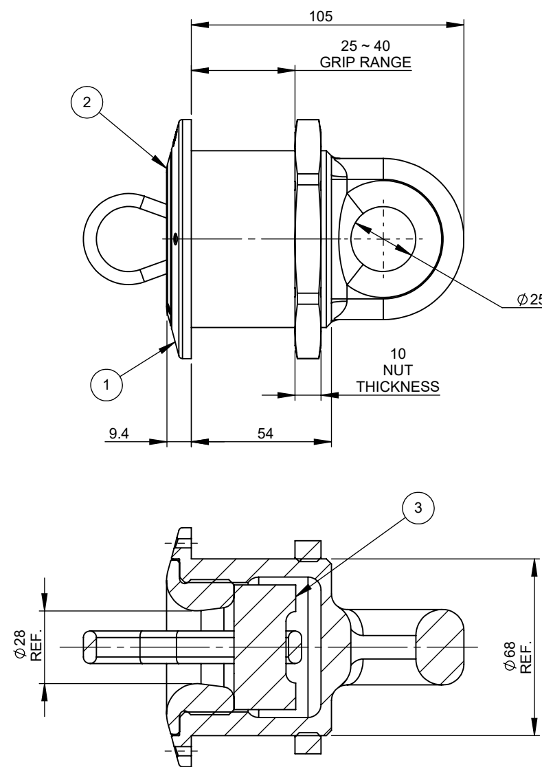
SECTION A-A
