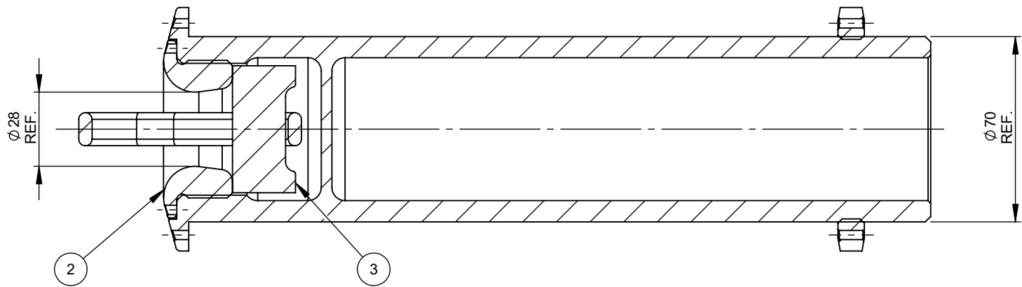
SECTION A-A
