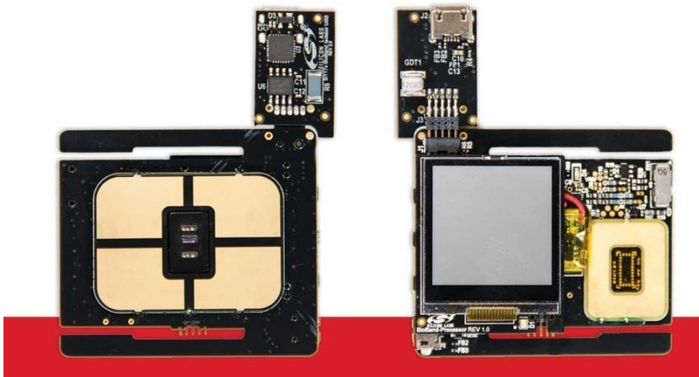
Bild 13. Die biometrischen Sensoren Si117X von Silicon Labs befinden sich in einem 28-Pin-LGA-Modul mit 3,7mm x 7mm. Ausserdem gibt es EKG- und PPF-Entwicklungs-Kits fürs Handgelenk. (Bild: Pressebild Silicon Labs)
