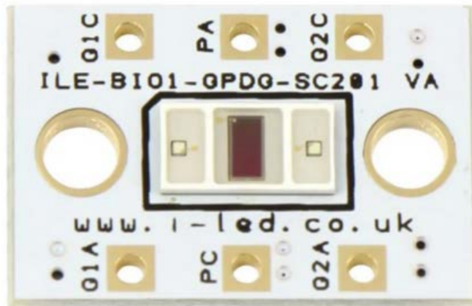
Bild 10. Das SFH7070 enthält zwei grüne LEDs mit 530nm und einen Detektor mit einer spektralen Empfindlichkeit im Bereich von 402 bis 694nm. (Bild: RS Components)
