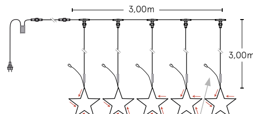
câble de suspension et sécurisation
