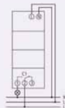
Schéma de raccordement
