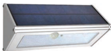
APPLIQUE SOLAIRE FIXE OU A DETECTION IP65, 3,2W, 1000lm, 4 modes de fonctionnement au choix
