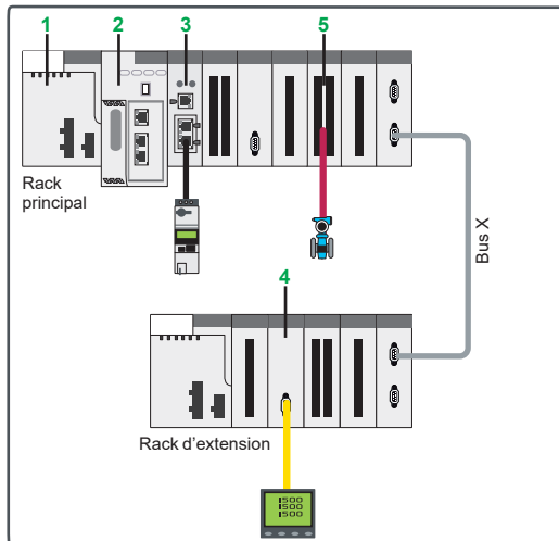
Architecture à bus de terrain intégrés : équipements distribués sur bus de terrain
