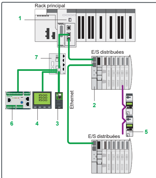
Architecture avec E/S distribuées : équipements distribués sur Ethernet avec DRS Modicon
