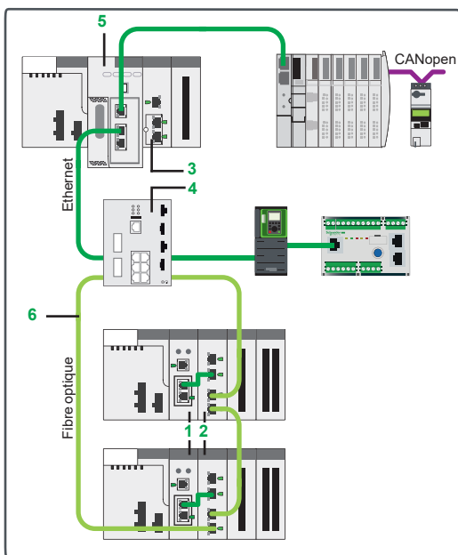
Architecture avec E/S distribuées + architecture avec E/S distantes
