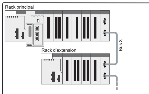
Architecture avec E/S locales : équipements sur E/S locales
