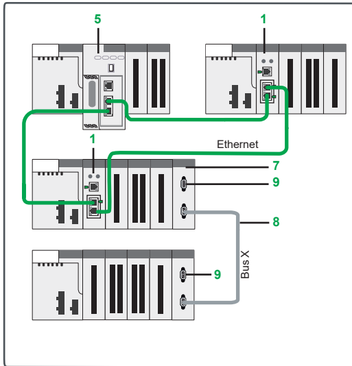
Architecture avec E/S locales + architecture avec E/S distantes
