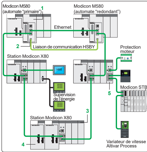
Architecture d'entrées/sorties décentralisées RIO
