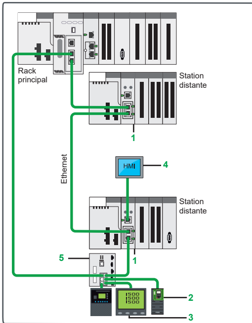
Architecture avec E/S distantes : équipements sur E/S distantes
