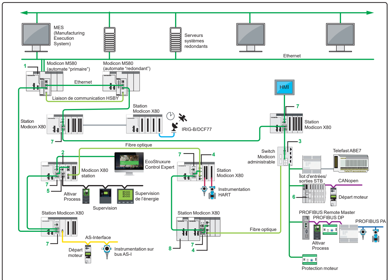
Exemple d'architecture complexe
