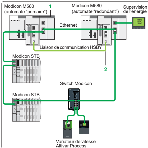
Architecture d'entrées/sorties distribuées DIO
