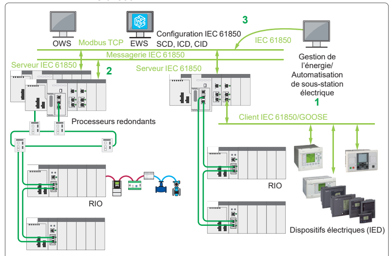
Différents services offerts par le module BMENOP0300
