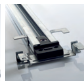
Fixation par embrochage et rotation (brevet FAAC)
