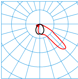
Jovie 50I-AM2L-SLR1/6800-740 6G1 ET (CLO end value) TX300860 ■ C0 - C180 ■ C90 - C270 DIN 5040: A40 UTE: 1,00 F CEN Flux Code: 47 91 100 100 100
