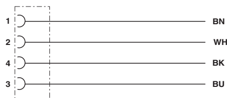
Affectation des contacts du connecteur femelle M12
