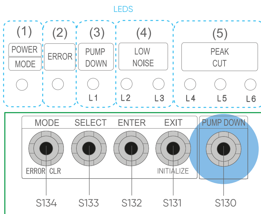
Boutons poussoirs
