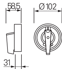
Schaltvorsatz GHG264
