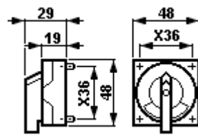
Schaltevorsatz Ex 23
