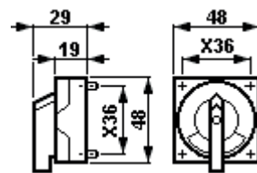
Schaltvorsatz Ex 23
