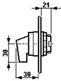
Schaltvorsatz Ex 41
