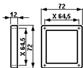
Messinstrumentenvorsatz M 72
