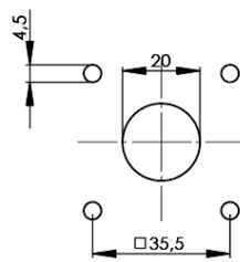
Bohrbild Schaltevorsatz Ex 23
