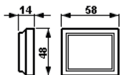
Messinstrumentenvorsatz M 45
