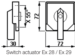
Switch actuator Ex 28 / Ex 29
