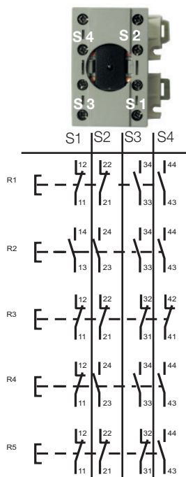
Actuator GHG41.11..R....; 2 x 2 pole
