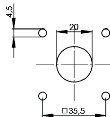
Bohrbild Schaltvorsatz Ex 23
