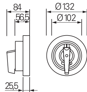
Schaltvorsatz GHG266
