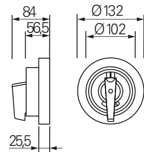
Schaltevorsatz GHG266
