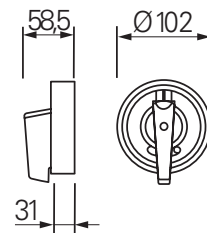
Schaltevorsatz GHG264
