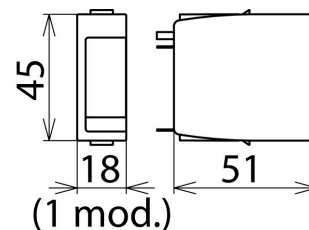
Dimensions DR MOD 30
