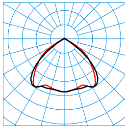
LightP G2 3P B-B-B 6500-830 05 NO TX055803
