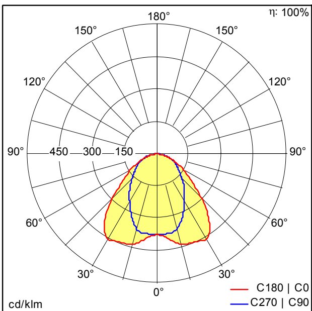
D41246AA_TECTON_C_LED5200-830_L1000_VWB_LDE_WH.Idt
