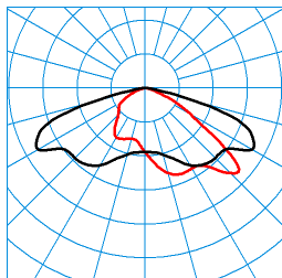
Jovie 70-AB7L-LRA/20000-740 24G1 ET (CLO end value) TX301188 ■ C0 - C180 ■ C90 - C270 DIN 5040: A30 UTE: 1,00 G CEN Flux Code: 35 73 97 100 100
