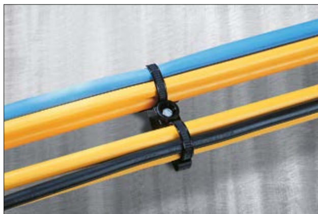
Lanière DSBS5 en application pour un routage en parallèle des câbles et faisceaux.
