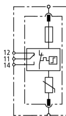
Schéma de principe du circuit DG S CI 440 FM
