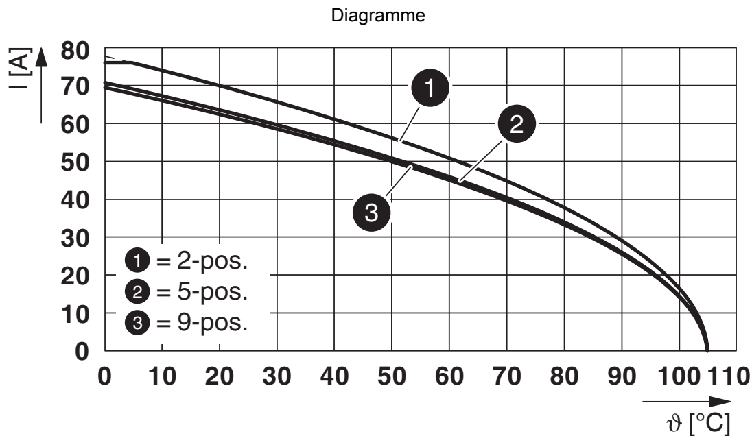
Type : SPC 16/...-STF-10,16 avec PC 6-16/...-G1FU-10,16
