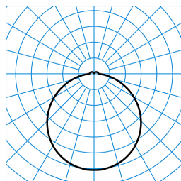
Olisq RWD2 DW 20-840 ETBLE +CAS IP54 + Olisq RWD2 ZDR 1/2 03 TX565961
