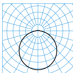
Olisq RWD2 DW 20-840 ETBLE +CAS IP54 + Olisq RWD2 C 01 TX565956
