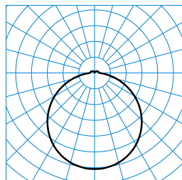
Olisq RWD2 DW 20-840 ETBLE +CAS IP54 + Olisq RWD2 ZDR 1/2 01 TX565960
