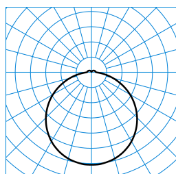
Olisq RWD2 DW 20-840 ETBLE +CAS IP54 + Olisq RWD2 ZDR 1/2 05 TX565962
