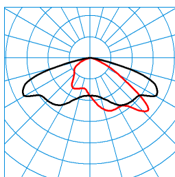
Jovie 70-AB7L-LR/13500-730 12G1 ET (CLO initial value) TX301223 ■ C0 - C180 ■ C90 - C270 DIN 5040: A30 UTE: 1,00 G CEN Flux Code: 34 72 96 100 100
