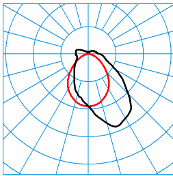
TugraHE 15 PAW 30-93/16ML-840 ET PC 23 (STAG10) TX425079 ■ C0 - C180 ■ C90 - C270 DIN 5040: B40 UTE: 0,86 E + 0,14 T CEN Flux Code: 48 77 92 86 100 13 32 64 14
