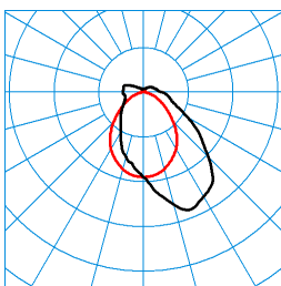
TugraHE 15 PAW 30-93/16ML-840 ET PC 23 (STAG14) TX425246 ■ C0 - C180 ■ C90 - C270 DIN 5040: B40 UTE: 0,86 E + 0,14 T CEN Flux Code: 48 77 92 86 100 13 32 64 14
