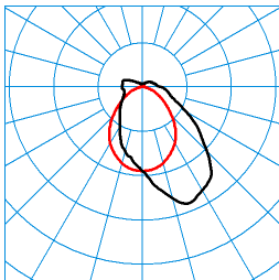
TugraHE 15 PAW 30-93/16ML-840 ET PC 23 (STAG13) TX425119 ■ C0 - C180 ■ C90 - C270 DIN 5040: B40 UTE: 0,86 E + 0,14 T CEN Flux Code: 48 77 92 86 100 13 32 64 14
