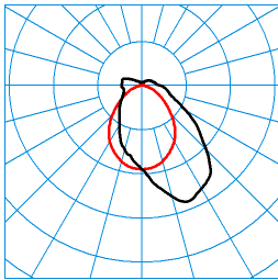
TugraHE 15 PAW 30-93/16ML-840 ET PC 23 (STAG11) TX425162 ■ C0 - C180 ■ C90 - C270 DIN 5040: B40 UTE: 0,86 E + 0,14 T CEN Flux Code: 48 77 92 86 100 13 32 64 14
