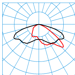
LnPlus 40-AB7L-LR/8200-740 8G1 ET (CLO initial value) TX377006 ■ C0 - C180 ■ C90 - C270 DIN 5040: A30 UTE: 1,00 G CEN Flux Code: 35 73 98 100 100
