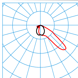
Jovie 50I-AM2L/4200-740 4G1 ETDD TX195492 ■ C0 - C180 ■ C90 - C270 DIN 5040: A40 UTE: 1,00 F CEN Flux Code: 47 91 100 100 100
