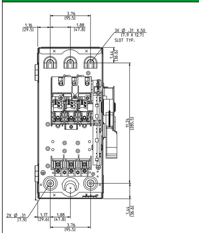
Type 1 30 A 240 V / 600 V Type 60 A 240 V
