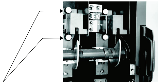
Tapón aislante
