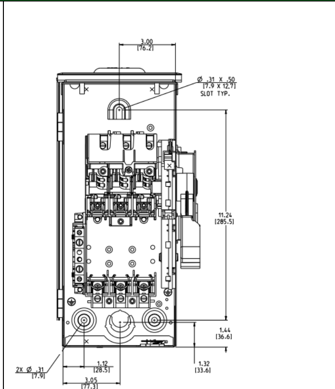
Tipo 3R 30 A 240 V/600 V Tipo 60 A 240 V
