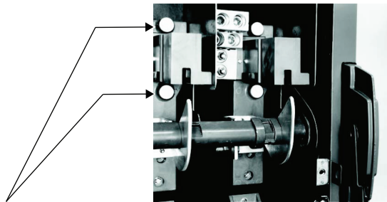
Obturbateur isolant
