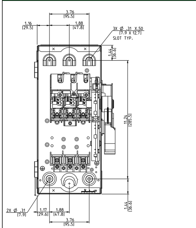
Tipo 1 30 A 240 V/600 V Tipo 60 A 240 V
