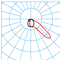
Jovie 50I-AM2L-LRA/5100-730 6G1 ET TX195509 ■ C0 - C180 ■ C90 - C270 DIN 5040: A40 UTE: 1,00 F CEN Flux Code: 47 91 100 100 100
