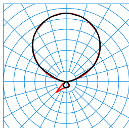
Luceos S-T PAW-IL 300-830 ETDI 03+LLWP (LEO2) TX830346
