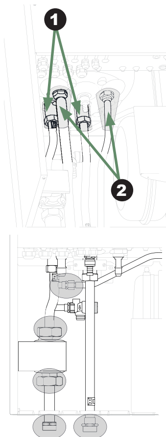
fig. 1 - Isolation thermique
