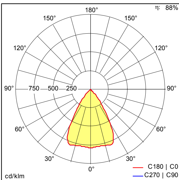
ST7932_N.Idt
