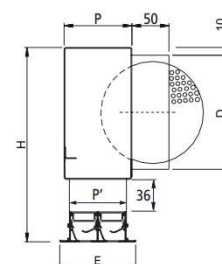
Diffuseur avec plénum
