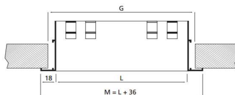
Coupe longitudinale du diffuseur seul
