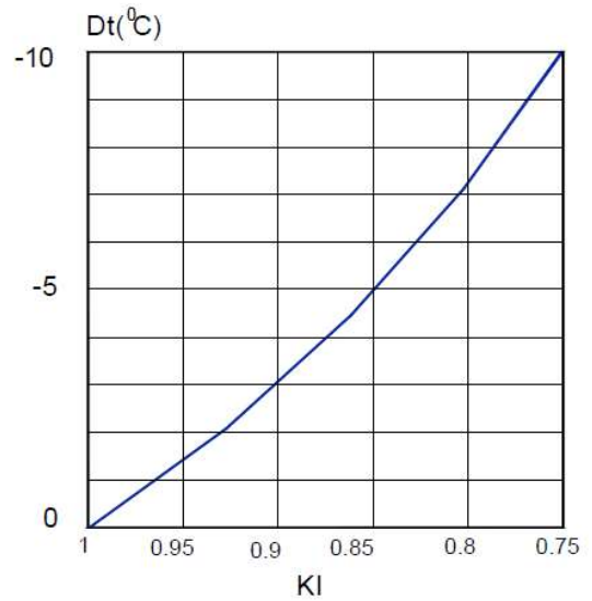
FACTEUR DE CORRECTION DE LA PORTÉE ( L_{0.2} ) Dt (-)
