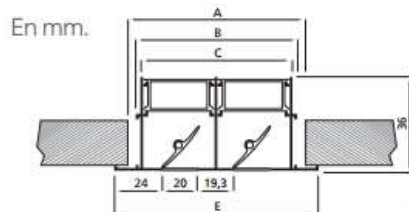
Coupe transversale du diffuseur seul
