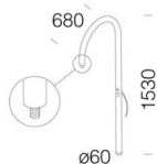
1473 Bras courbé
