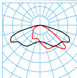
Jovie 70-AB7L-ML/75-150-740 12G1 ETDD (10000 lm) TX068726 ■ C0 - C180 ■ C90 - C270 DIN 5040: A30 UTE: 1,00 G CEN Flux Code: 34 72 96 100 100
