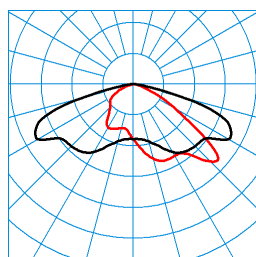
Jovie 70-AB7L-ML/75-150-740 12G1 ETDD (7500 lm) TX068728 ■ C0 - C180 ■ C90 - C270 DIN 5040: A30 UTE: 1,00 G CEN Flux Code: 34 72 96 100 100
