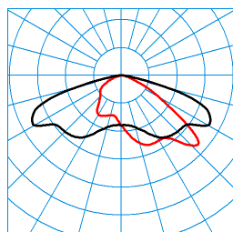
Jovie 70-AB7L-ML/75-150-740 12G1 ETDD (15000 lm) TX068727 ■ C0 - C180 ■ C90 - C270 DIN 5040: A30 UTE: 1,00 G CEN Flux Code: 34 72 96 100 100
