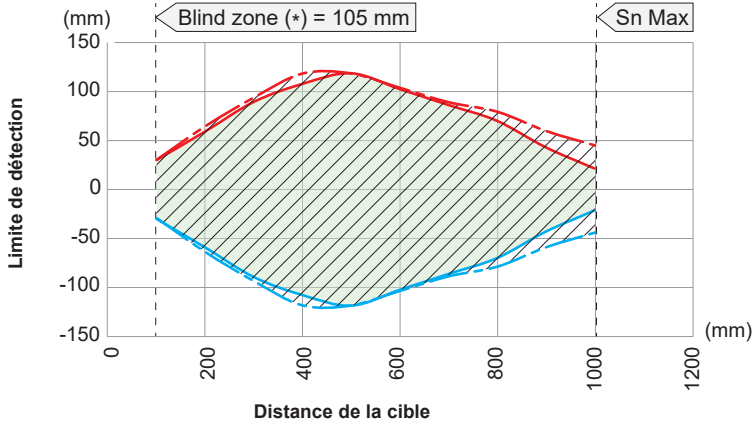
Courbe de détection avec barre ronde
