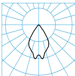
InperiaLP C05 BR19 1000-840 01 + RG-PC TX373888 ■ C0 - C180
