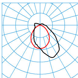
TugraHE 18 PAW 65-100/16ML-830 ET PC 23 (STAG13) TX425226 ■ C0 - C180 ■ C90 - C270 DIN 5040: B40 UTE: 0,86 E + 0,14 T CEN Flux Code: 48 77 92 86 100 13 32 64 14
