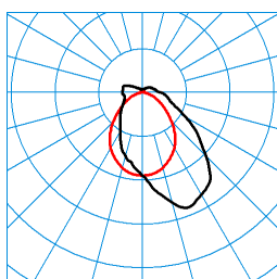
TugraHE 18 PAW 65-100/16ML-830 ET PC 23 (STAG14) TX425125 ■ C0 - C180 ■ C90 - C270 DIN 5040: B40 UTE: 0,86 E + 0,14 T CEN Flux Code: 48 77 92 86 100 13 32 64 14
