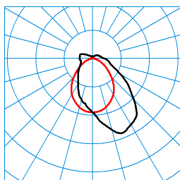
TugraHE 18 PAW 65-100/16ML-830 ET PC 23 (STAG11) TX425097 ■ C0 - C180 ■ C90 - C270 DIN 5040: B40 UTE: 0,86 E + 0,14 T CEN Flux Code: 48 77 92 86 100 13 32 64 14
