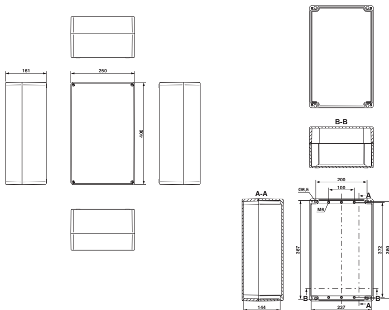
Dessin coté
