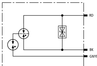
Schéma de principe du circuit DPI CD EXI 24 N
